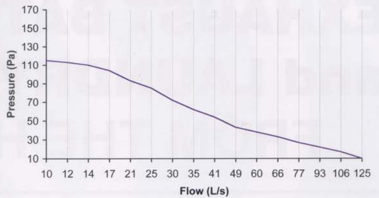
Fan Curve
